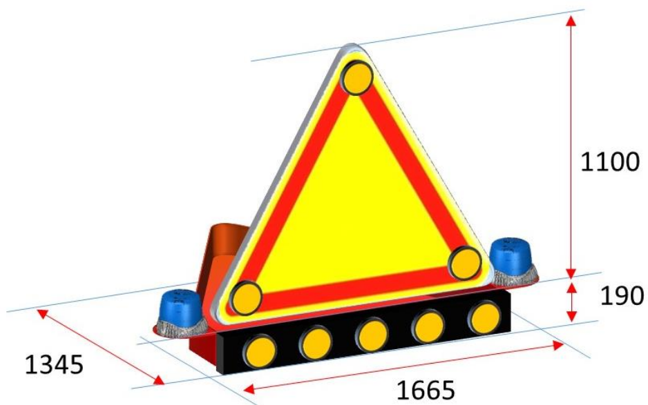
TRIANGLE 1250 : 50 kg
