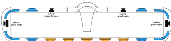
Modèle présenté : rampe VEGA avec sirène intégrée, défilement arrière (5 feux orange) et option vidéo
