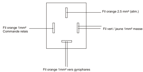
Détails relais gyrophares intérieurs
