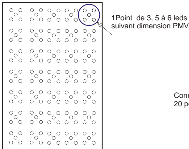
Vue avant carte a leds
