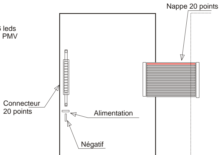
Vue arrière carte a leds
