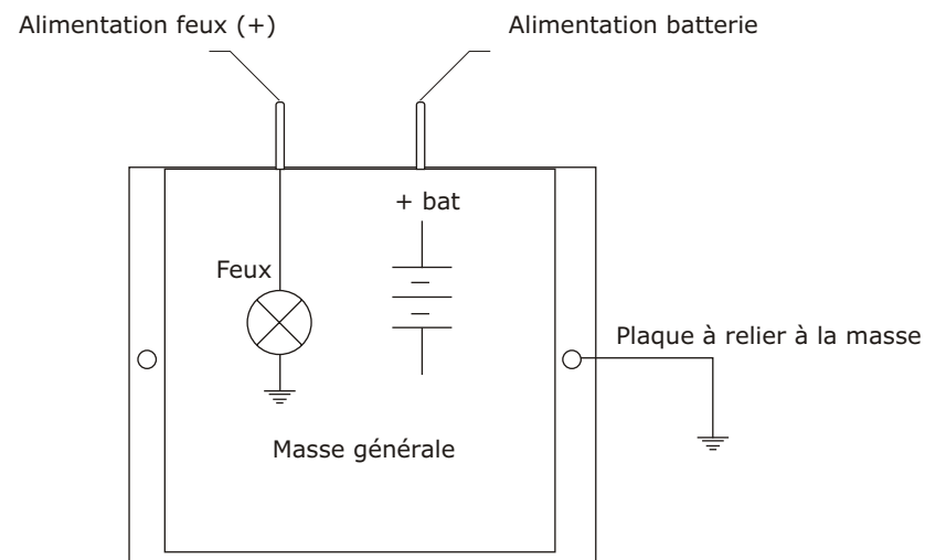
Centrale clignotante sorties 2 languettes
