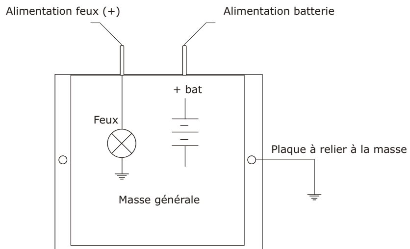
Centrale clignotante sorties 2 languettes
