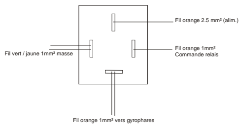
Détails relais gyrophares intérieurs
