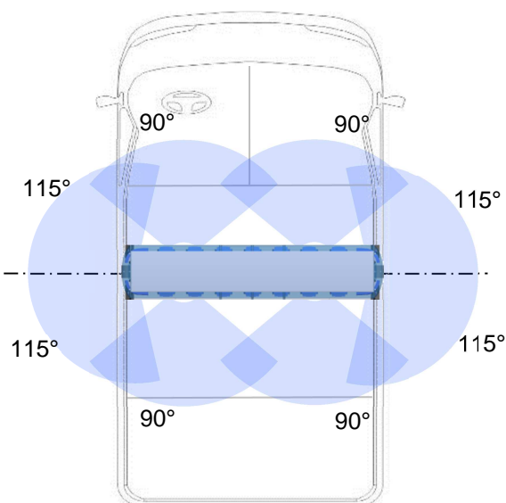
Rampe VEGA BF1
