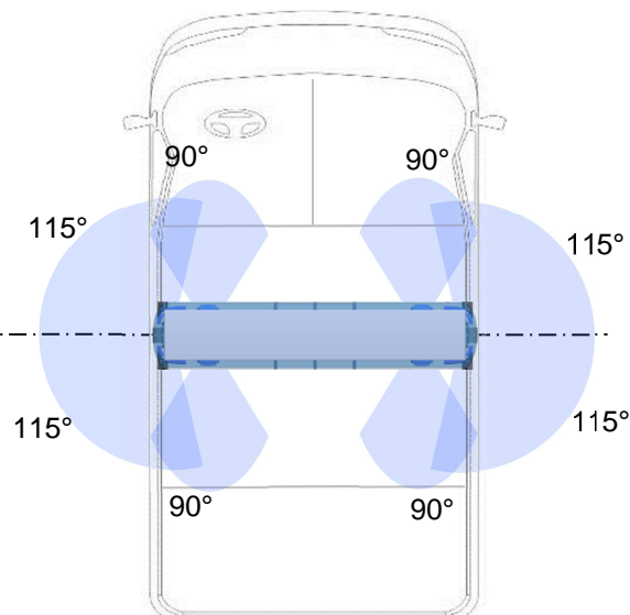
Rampe VEGA BF3
