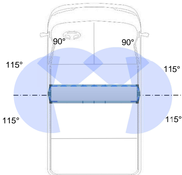
Rampe VEGA BF2
