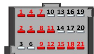
CONNECTEUR 21 POINTS
