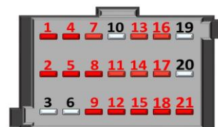
CONNECTEUR 21 POINTS
