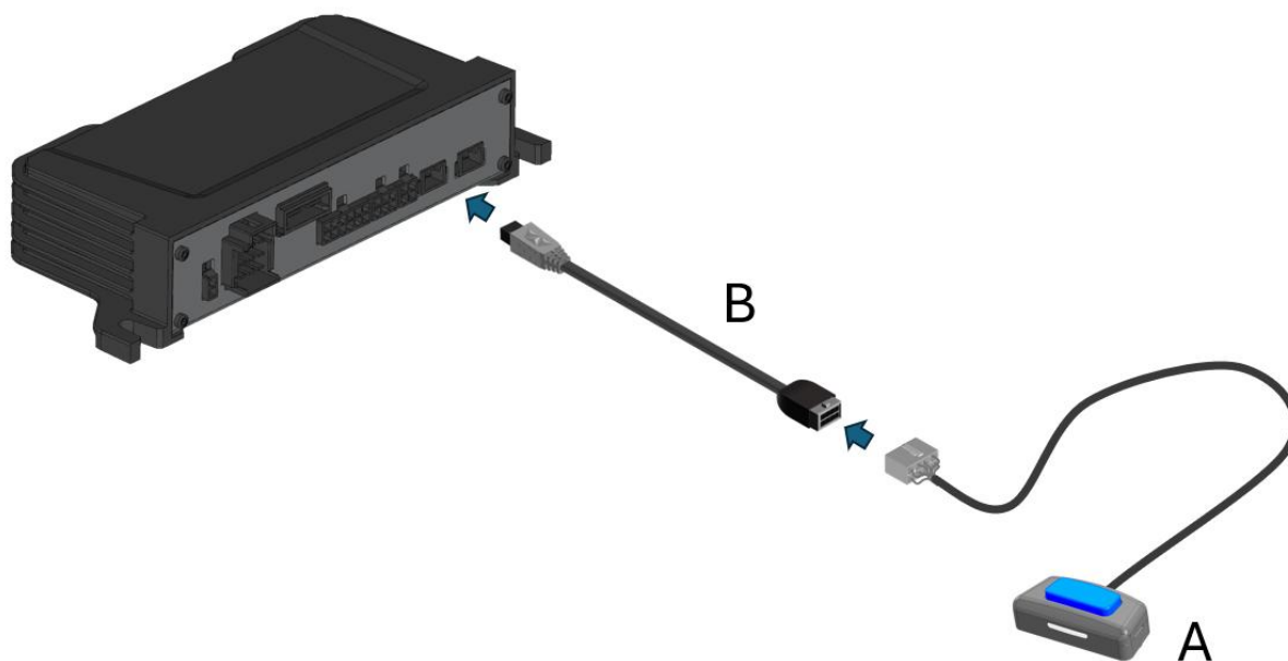
A. Bouton d'urgence H1 (30665)
